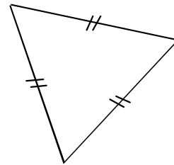
Le triangle équilatéral
