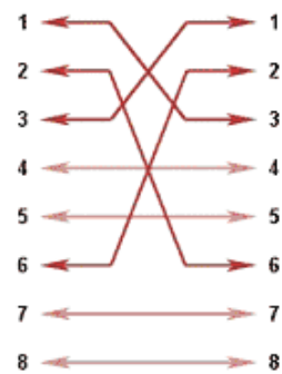
Câble croisé
