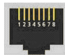
Numérotation des contacts prise vue de face
